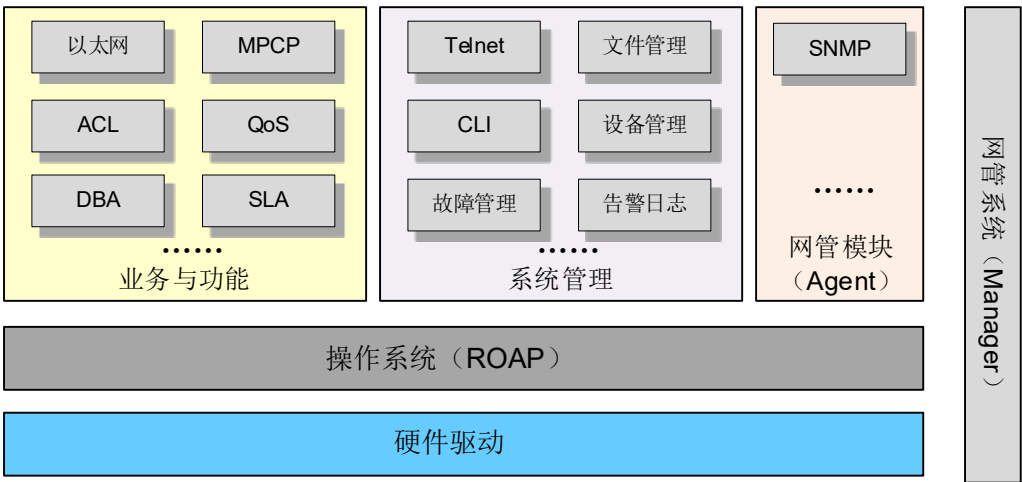
图 2-7 P7000 软件结构图
