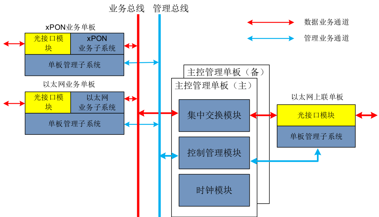
图 2-8 P7000 功能结构
