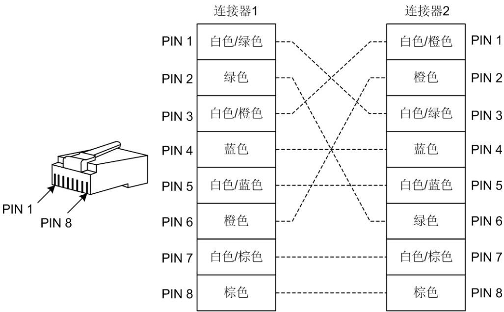
图 2-24 100Mbit/s 交叉网线接线图
