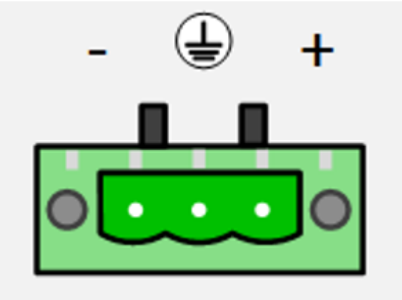
图 2-14 直流电源 2 模块
