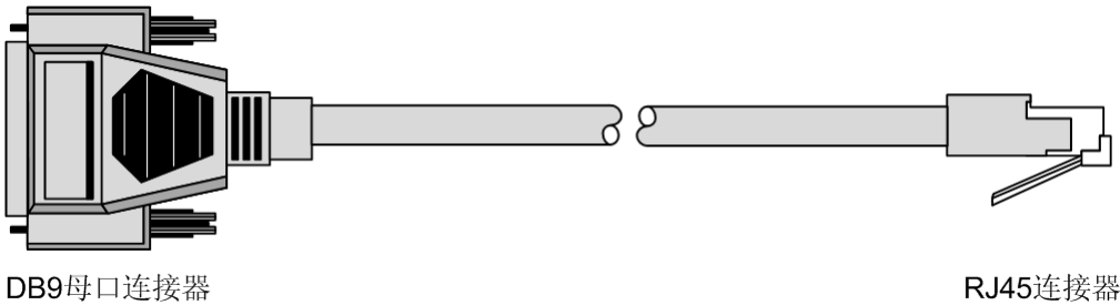
图 2-39 Console 线示意图
