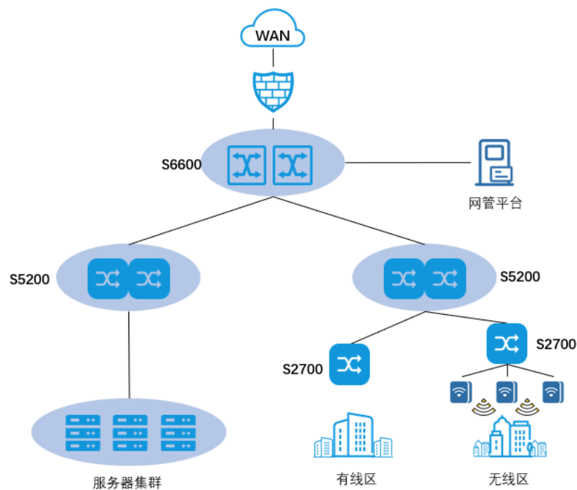
图 1-2 企业园区接入组网图
