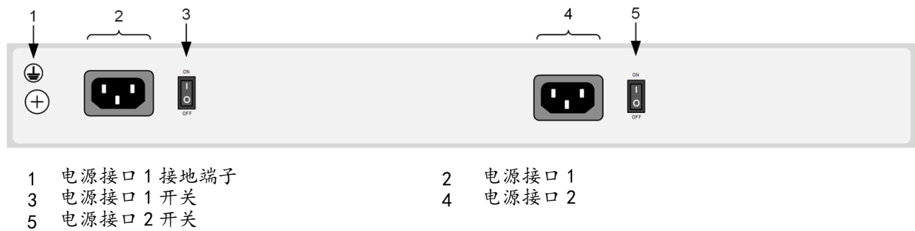
图 2-2 S2700 后面板外观
