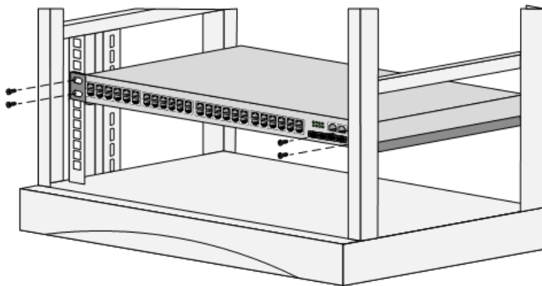
图 4-6 水平安装设备到机架
