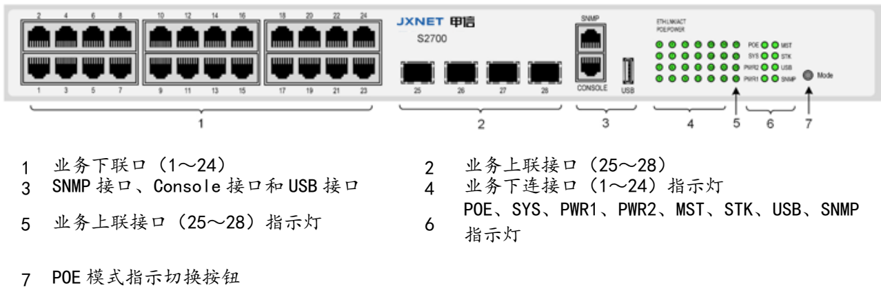
图 2-1 S2700 前面板外观
