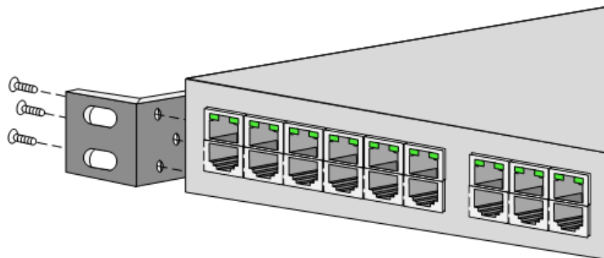
图 4-3 安装挂耳
