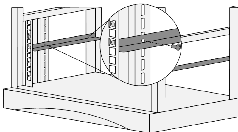
图 4-5 安装滑道
