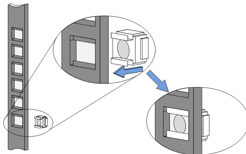
图 4-4 安装浮动螺母
