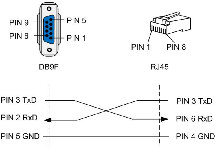
图 2-41 接线关系示意图
