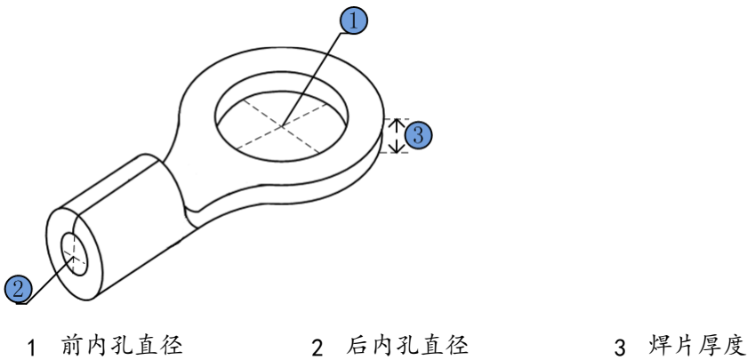
图 2-28 OT 端子示意图
