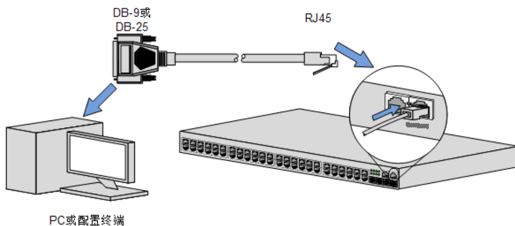
图 4-15 连接 Console 串口线
