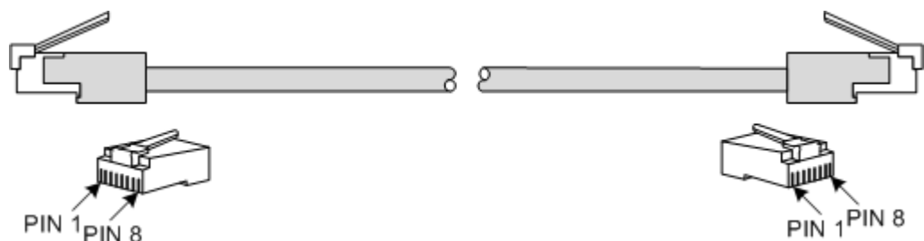
图 2-21 网线示意图
