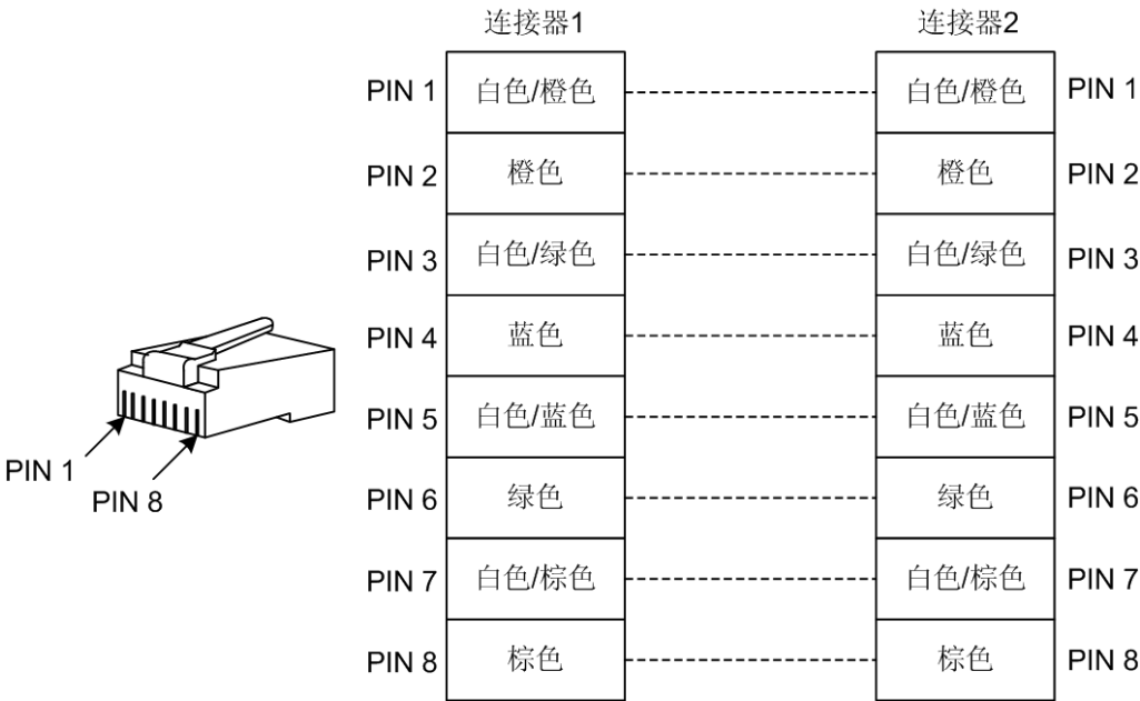
图 2-23 10/100/1000M 直通网线接线图
