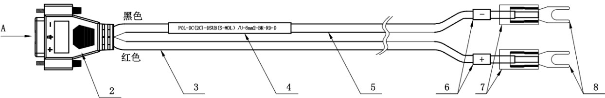
图 2-44 可插拔直流电源线示意图
