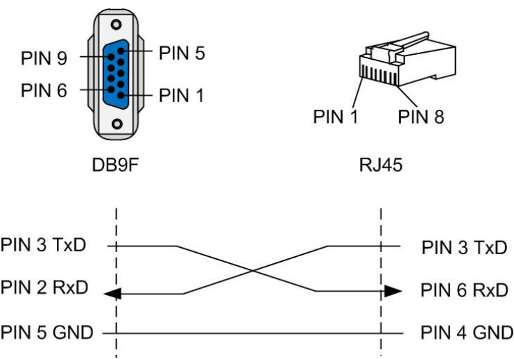
图 2-53 接线关系示意图
