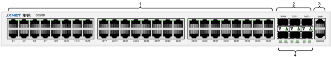
图 2-3 S5200-48T6X 前面板外观
