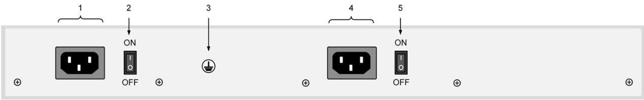
图 2-2 S5200-24T6X 后面板外观
