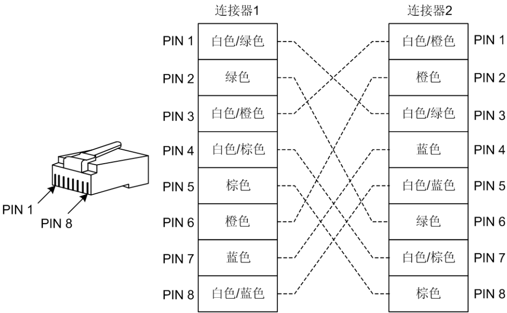
图 2-35 1000M 交叉网线接线图
