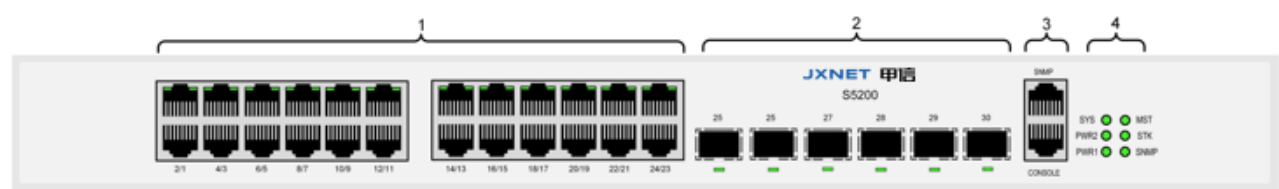
图 2-1 S5200-24T6X 前面板外观
