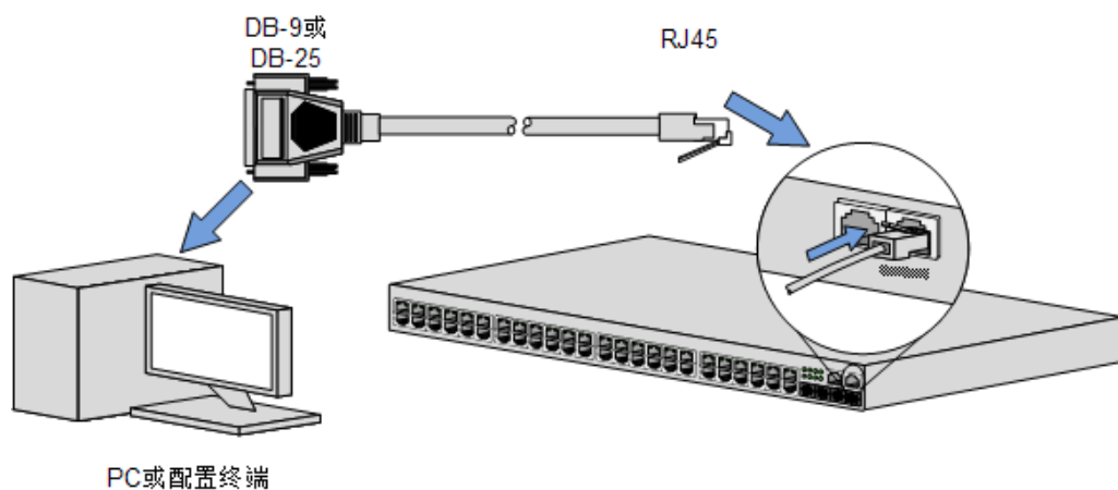
图 4-17 连接 Console 串口线
