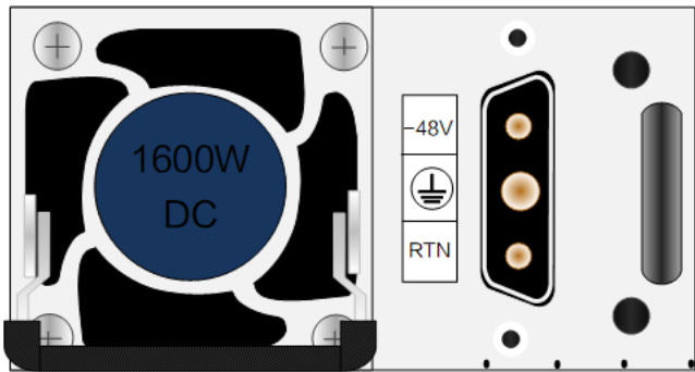
图 2-26 PoE 款型可插拔直流电源模块
