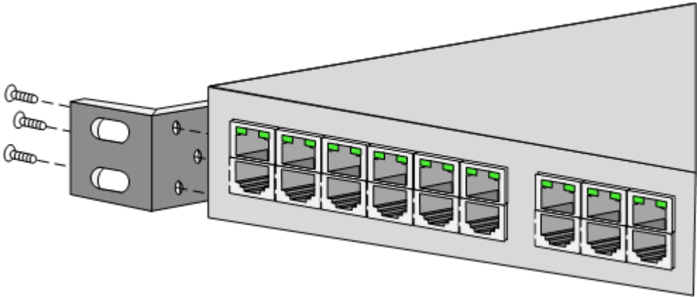
图 4-3 安装挂耳
