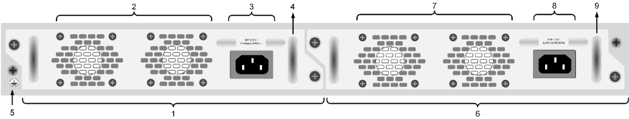
图 2-6 S5200-24S8T6X 后面板外观
