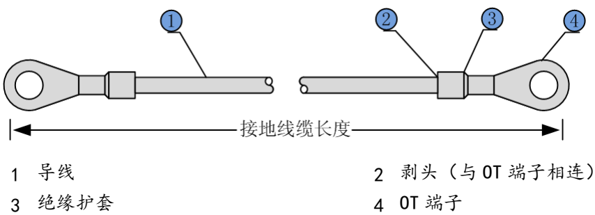
图 2-37 接地线缆示意图
