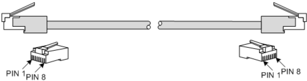
图 2-31 网线示意图
