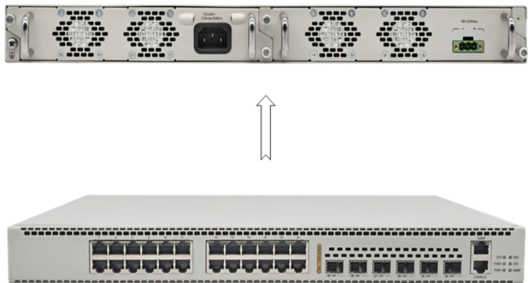
图 2-62 风扇 2 示意图
