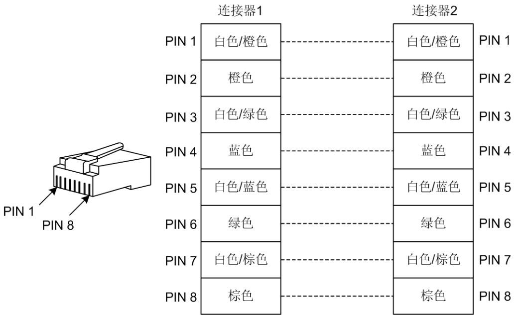
图 2-33 10/100/1000M 直通网线接线图
