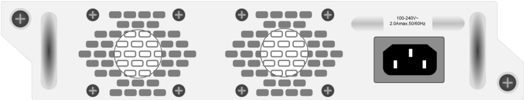
图 2-22 可插拔交流电源模块
