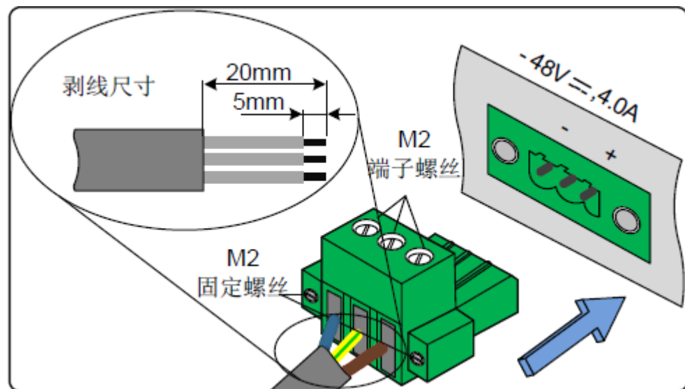
图 4-14 连接可插拔直流电源线缆
