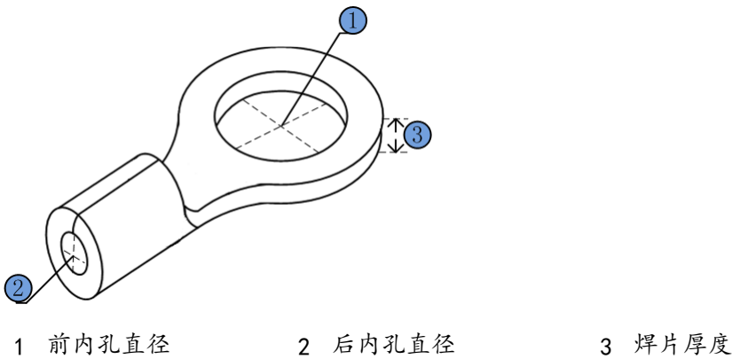
图 2-38 OT 端子示意图
