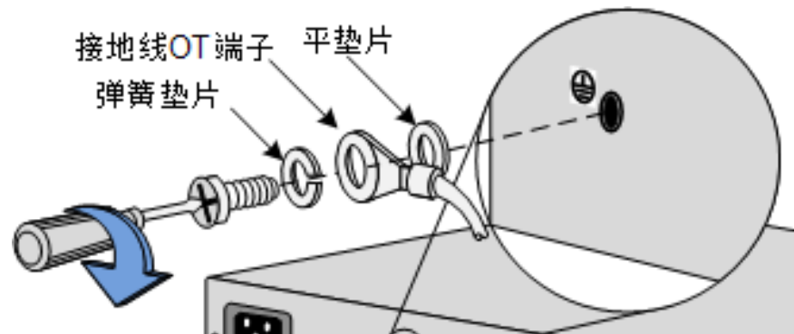
图 4-10 连接接地线缆
