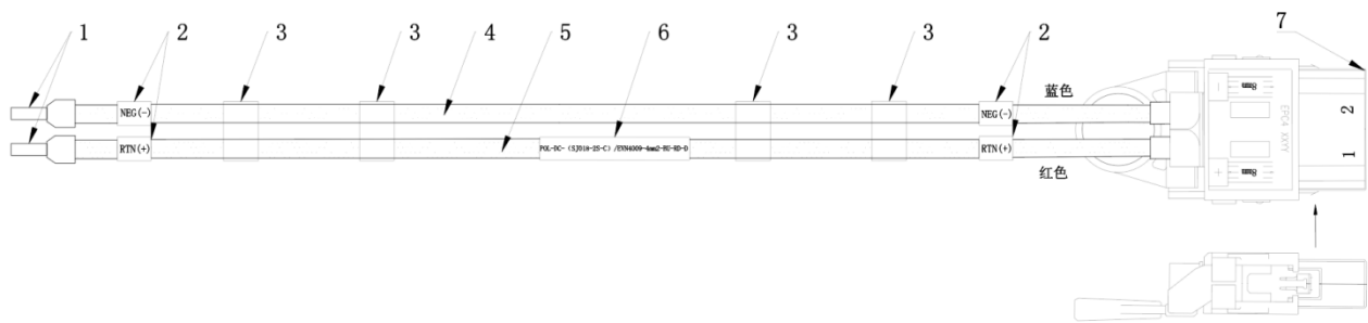
图 2-37 直流电源线示意图
