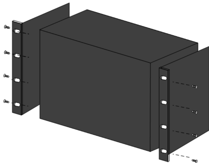
图 4-4 安装挂耳
