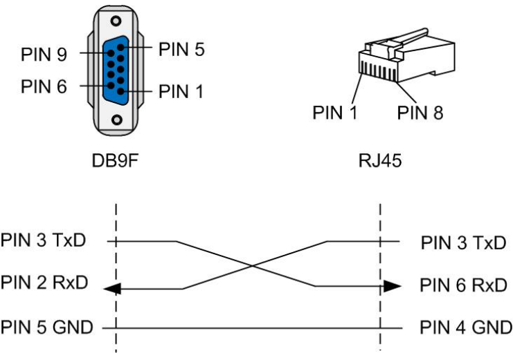
图 2-42 接线关系示意图
