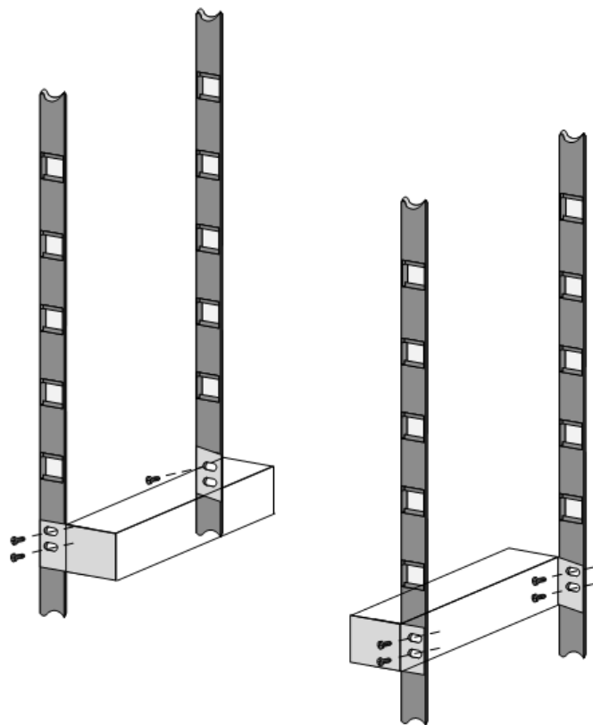
图 4-3 安装滑道
