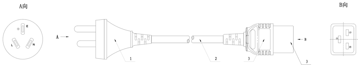
图 2-39 交流电源线示意图
