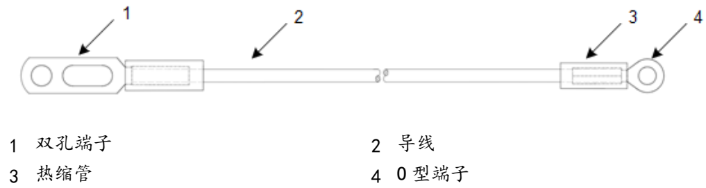
图 2-35 接地线缆示意图
