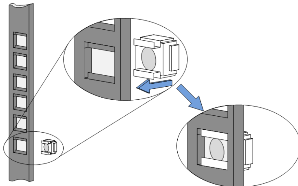
图 4-5 安装浮动螺母
