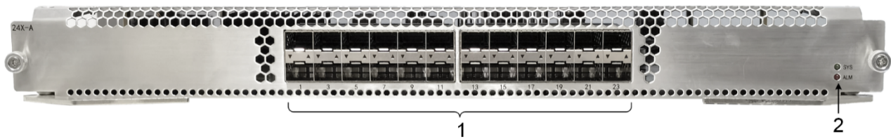
1 10GE SFP+接口及指示灯（1~24） 2 SYS、ALM 指示灯
