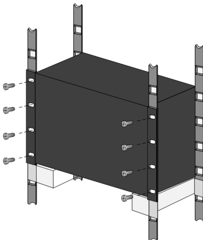
图 4-6 水平安装设备到机架
