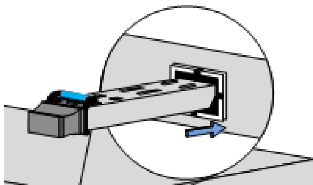
图 4-7 插入 SFP 光模块
