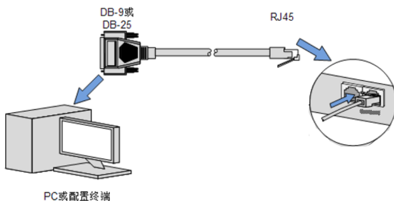
图 4-17 连接 Console 串口线
